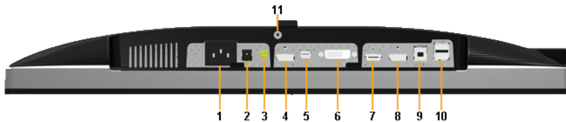
Vista inferior sin soporte de monitor
